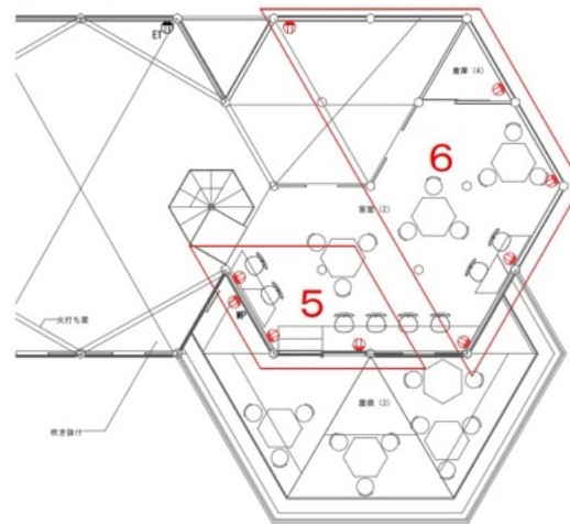
2階平面図
