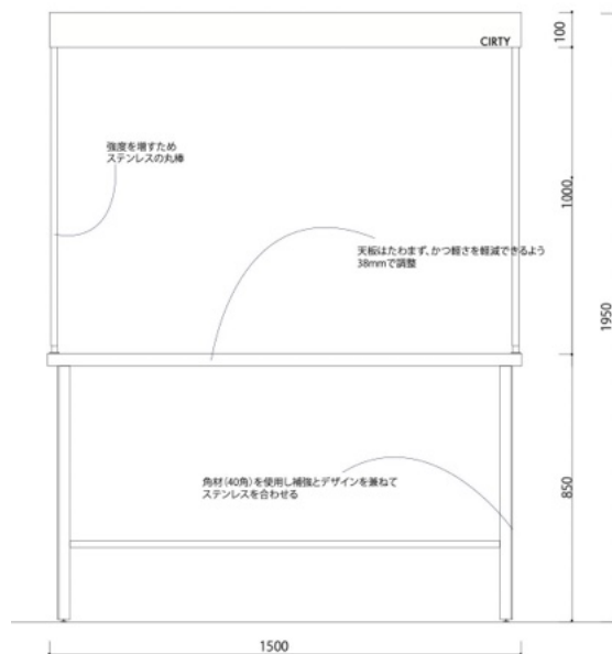
姿図 1/10
